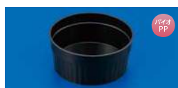
IR76-110H ●76パイ×33 ●バイオPP ●容量 110cc ●袋25/ケース500
